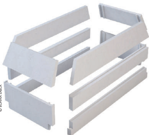
Exemple de caveau préfabriqué en panneaux assemblés
