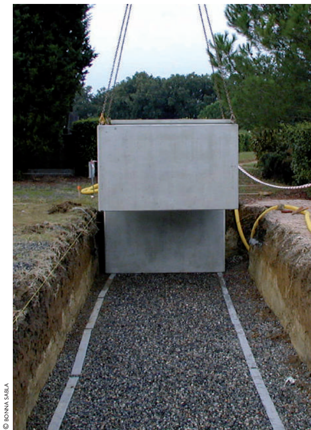
Caveau posé sur longrines avec sous couche drainante
